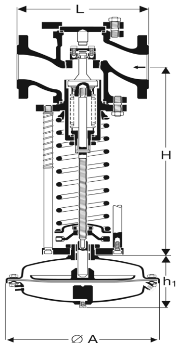
Перепускной клапан SelfAct 5601
